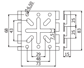
H64 / H105
